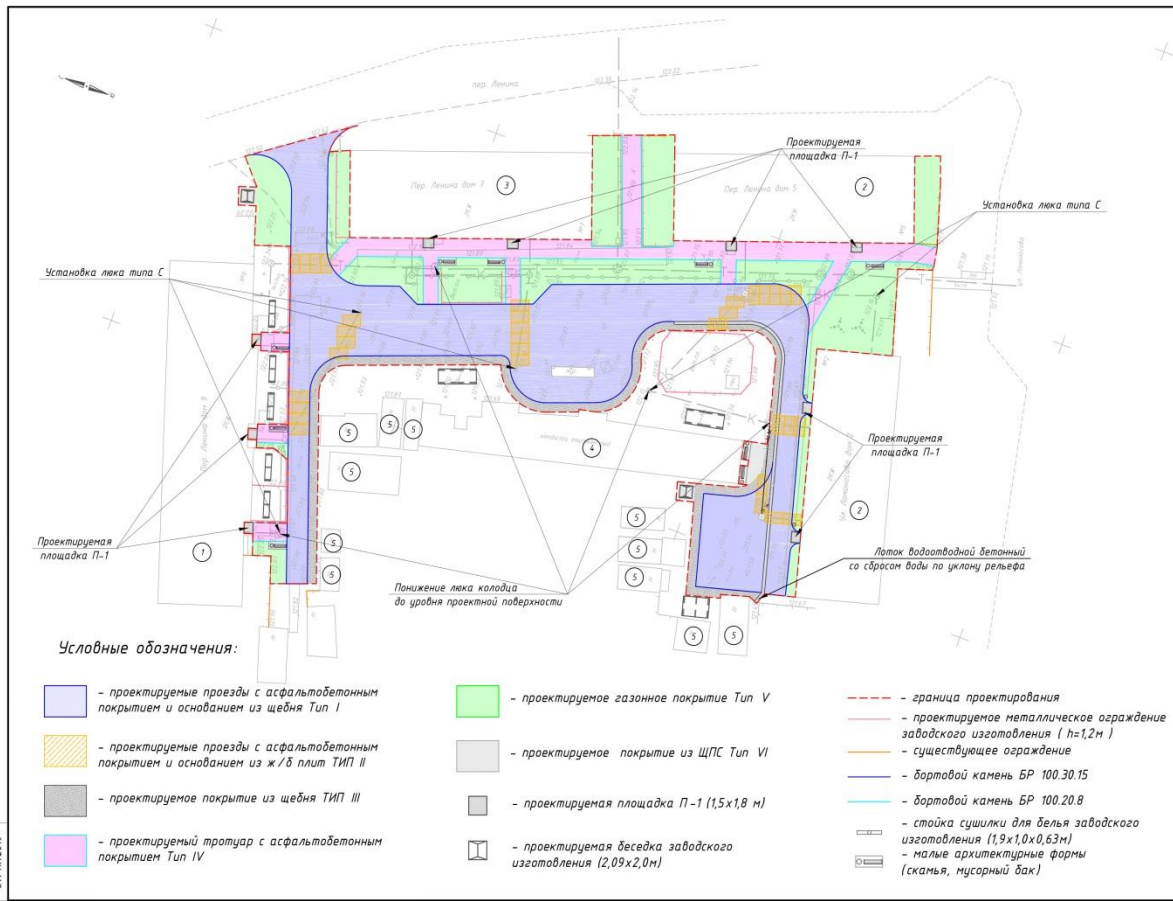
схема генерального плана
